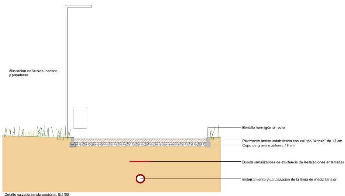
Detalle del plano de ordenación OD-02 del PERIM
