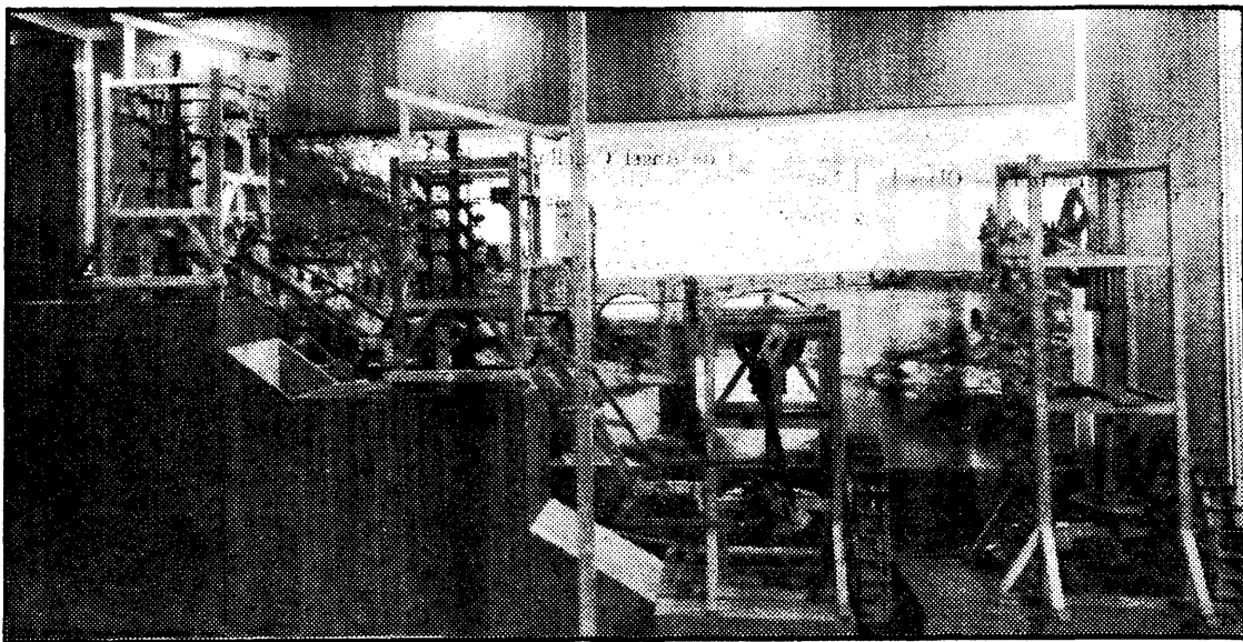
Maqueta del artificio de Juanelo que se guarda en el Palacio de la Diputación Provincial de Toledo
