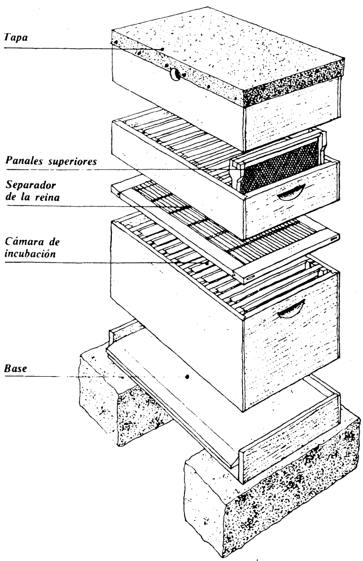
Esquema de la colmena y forma de colocar sus partes
