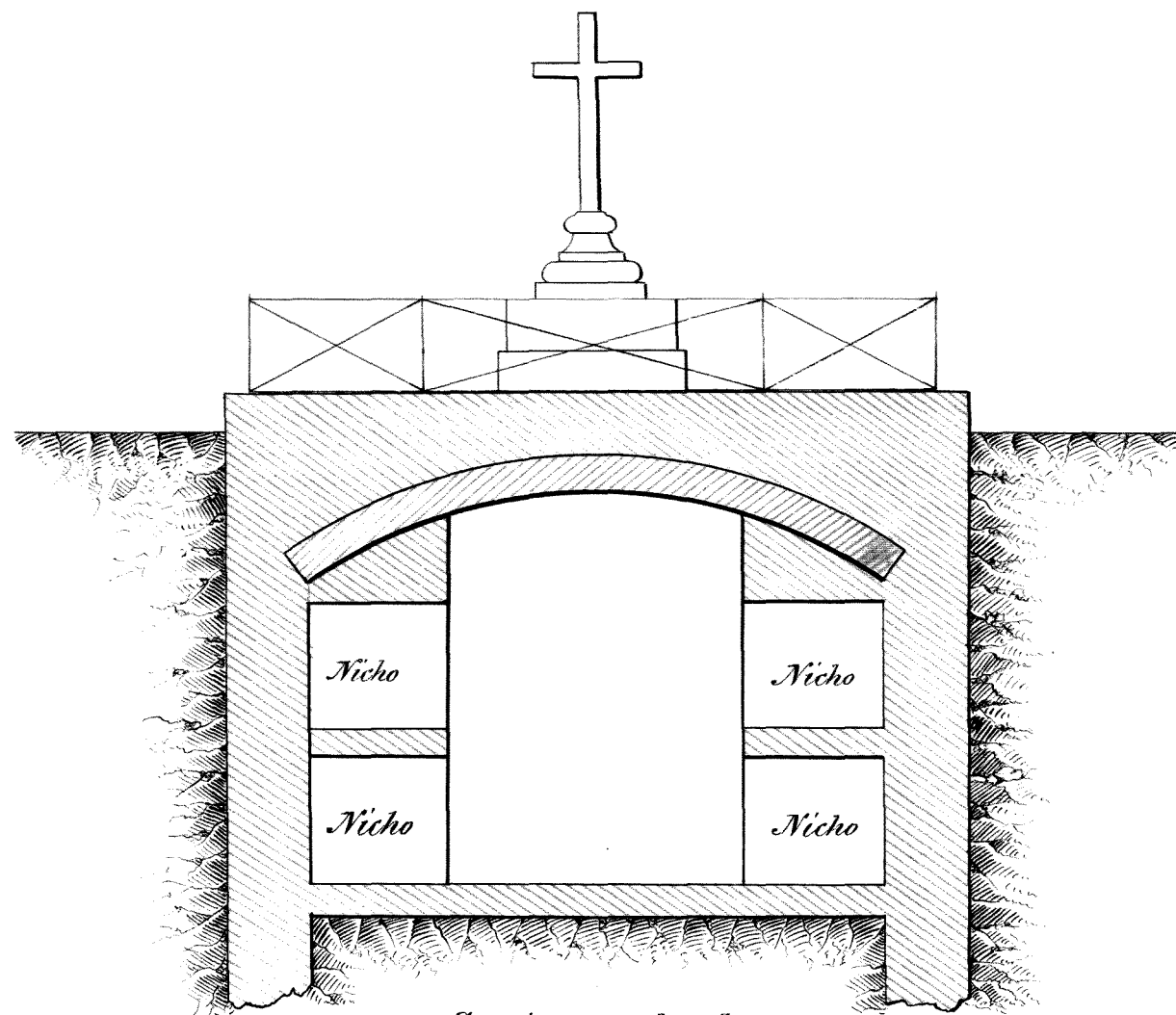
Sección y alzado.
