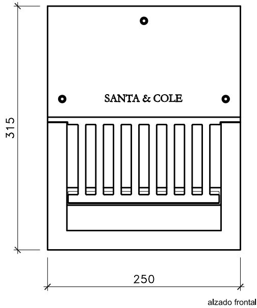
alzado frontal
