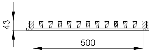
Sección AA'
